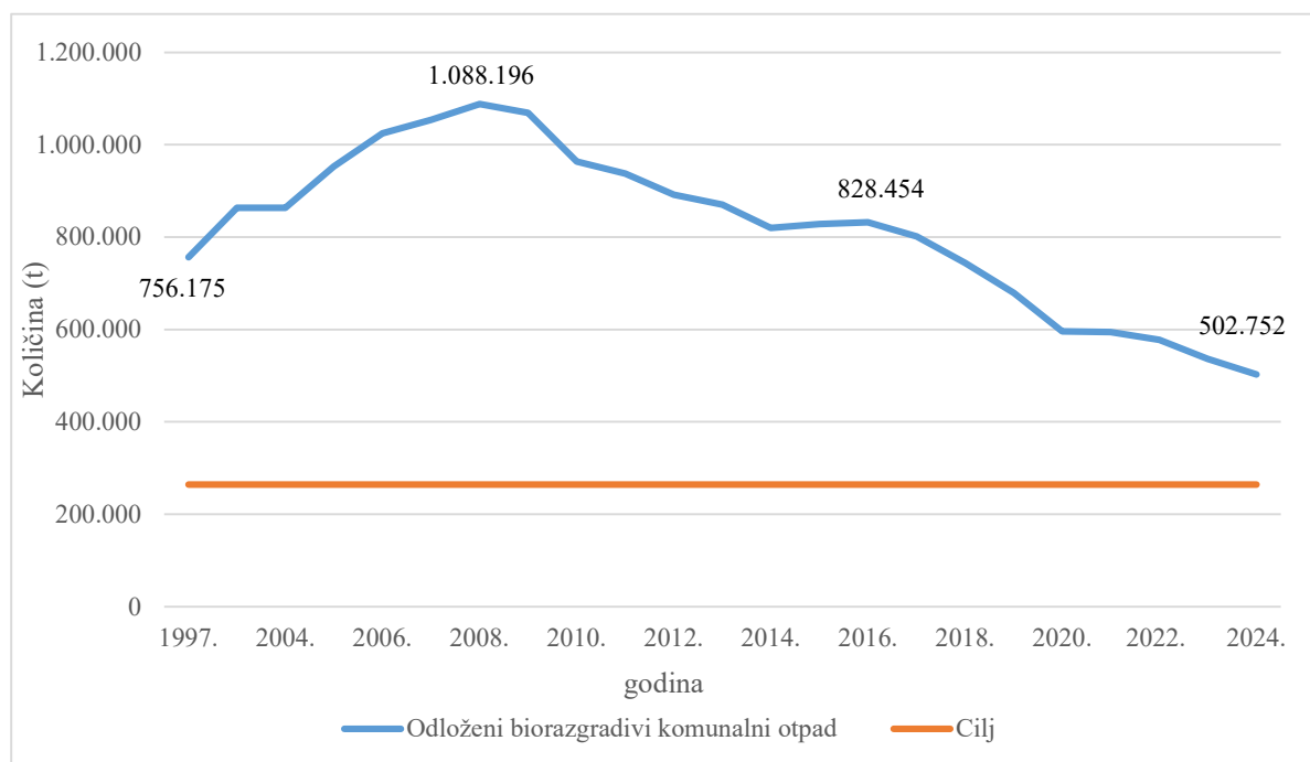
Slika 1. Odlaganje biorazgradivog komunalnog otpada u RH u razdoblju od 1997. do 2024. godine u odnosu na propisani cilj
