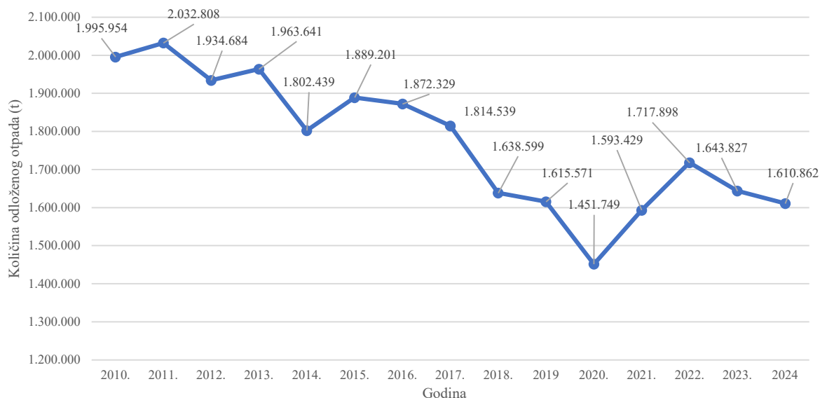
Slika 2. Odlaganje otpada u RH u razdoblju od 2010. do 2024. godine
